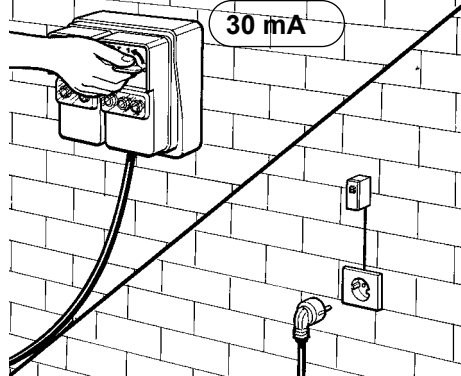
Tilslutning vandcirkulationen.
