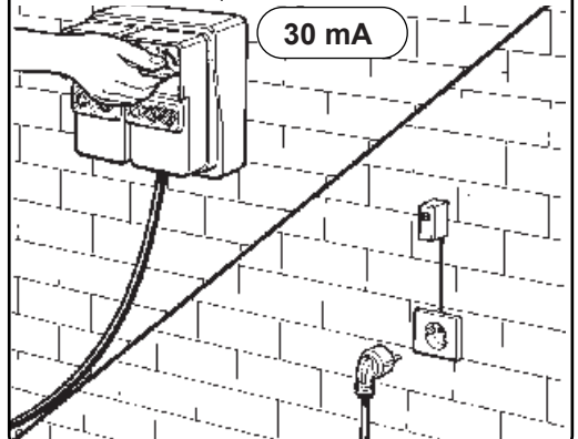
Branchement électrique.
