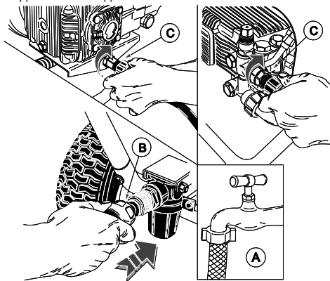
Подключение воды.
