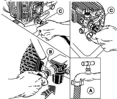
Ligação à rede hídrica.
