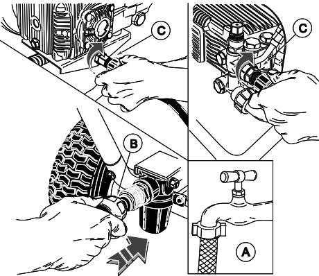
Wasseranschluß
