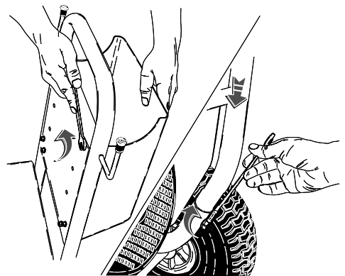
Montage de la poignée.
