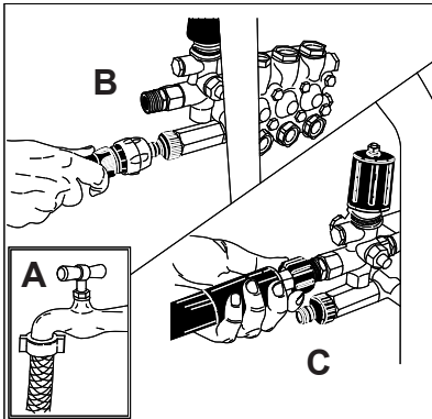
Подключение воды.
