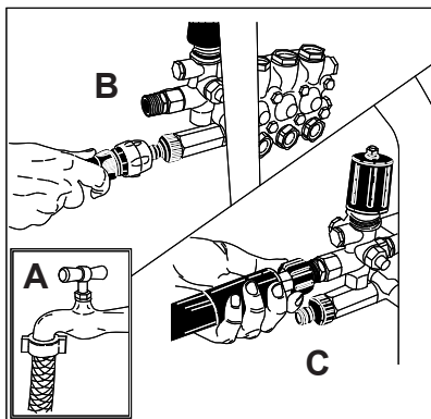
Wasseranschluß.
